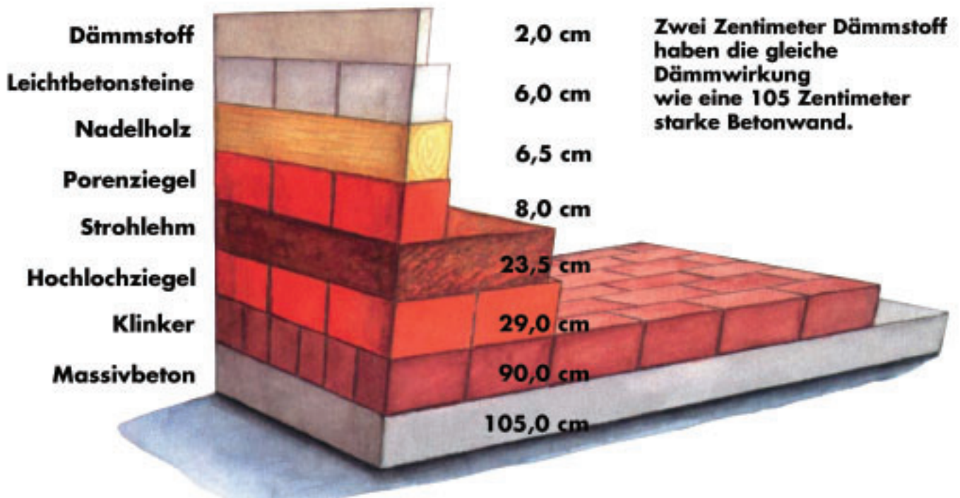
Dämmvermögen von Baustoffen
