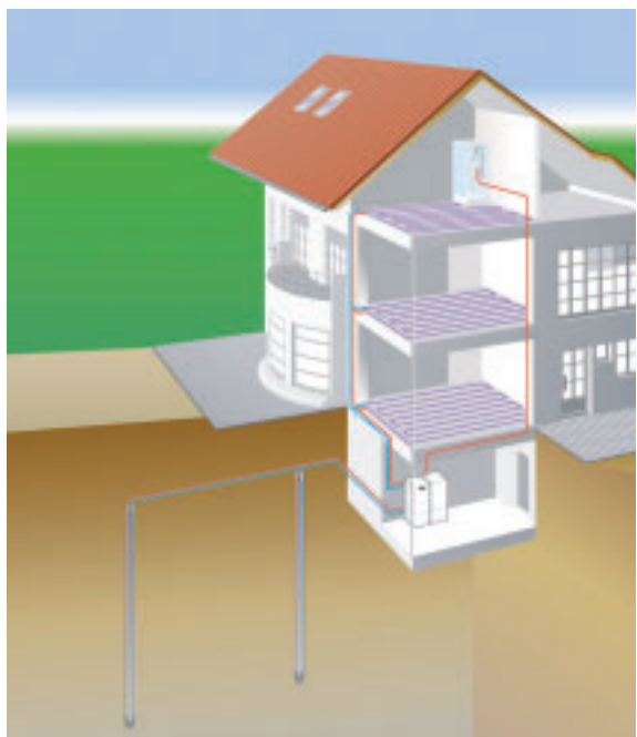
Schema einer Wärmepumpe mit Erdsonden (links) und mit Erdkollektor (rechts). Beide Wärmepumpen nutzen Erdwärme. Quelle: Max Weishaupt GmbH
