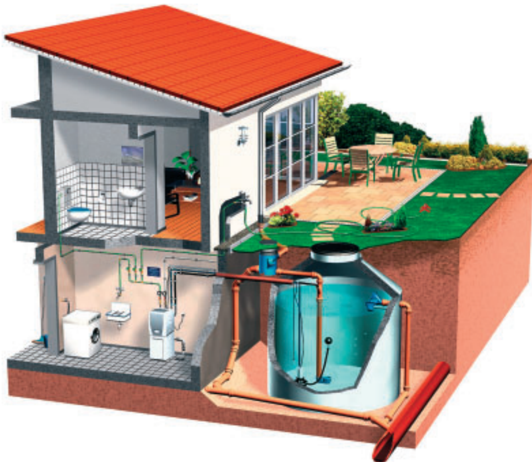
Schematische Darstellung der Regenwassernutzung
