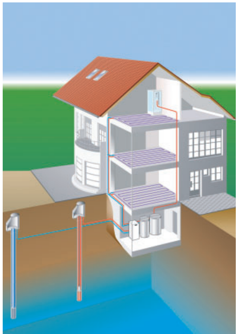
Schema einer Wärmepumpe mit Förder- und Schluckbrunnen. Diese Pumpe nutzt die Wärme des Grundwassers. Quelle: Max Weishaupt GmbH
