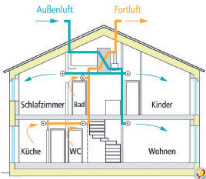
Kontrollierte Wohnungslüftung
