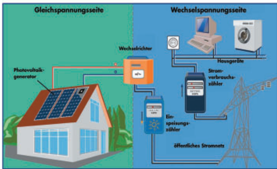
Funktionsprinzip einer Photovoltaik-Anlage
